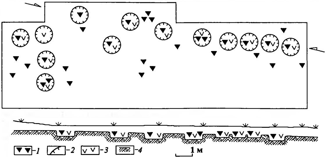
Рис.3. План та переріз „вовчих ям” з посаду Ленківців на Пруті (за Б. Тимощуком) 1 – залізні шлаки; 2 – контури ями; 3 – вугілля; 4 – материк
