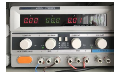
Блок живлення HT3005PB
